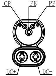
插头触头布置图
